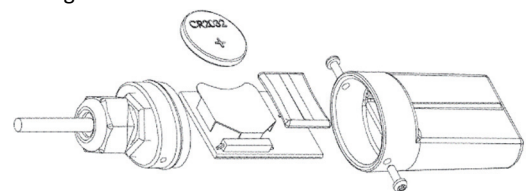
Batteriewechsel
